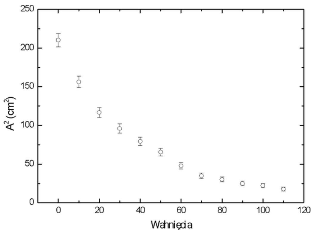
Rysunek 2: Zmierzona amplituda drgań wahadła bez płytki.
