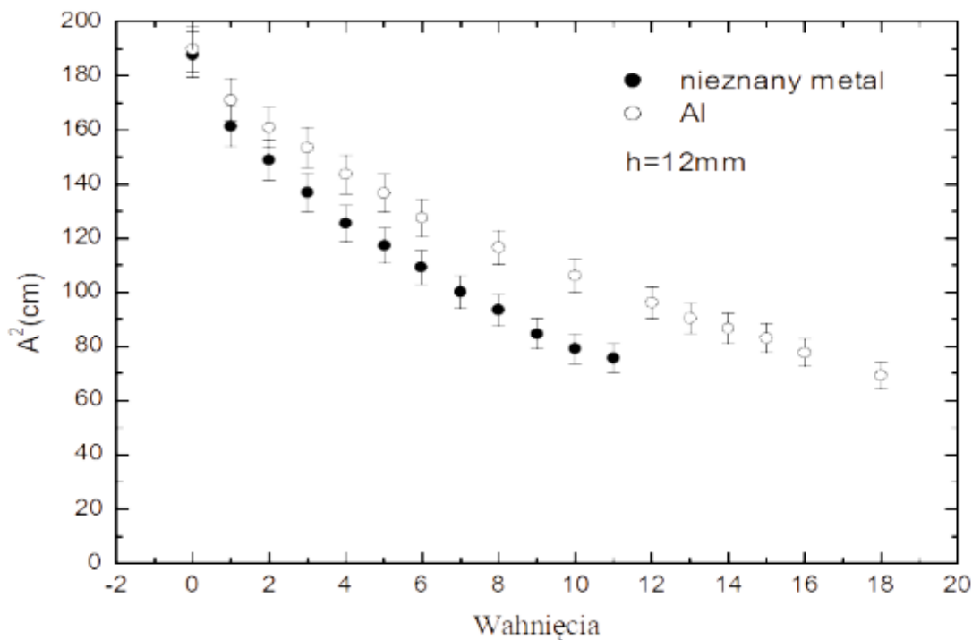
Rysunek 4: Zmierzona amplituda drgań wahadła z płytką aluminiową i tą z nieznanego metalu.
