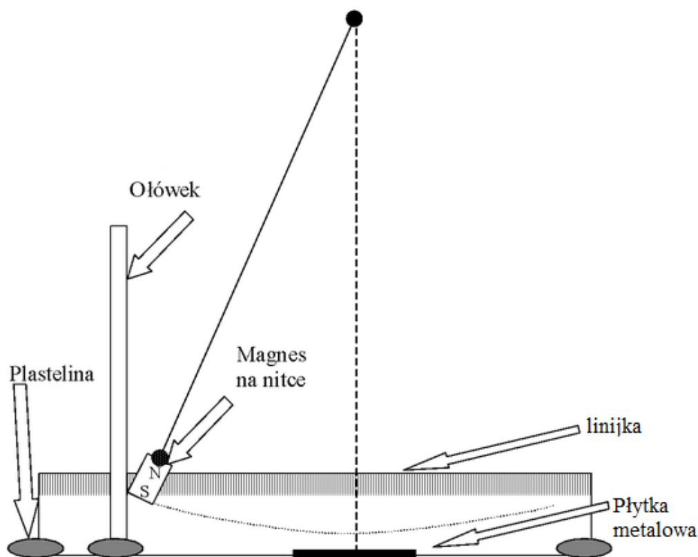
Rysunek 1: Schemat układu pomiarowego.
