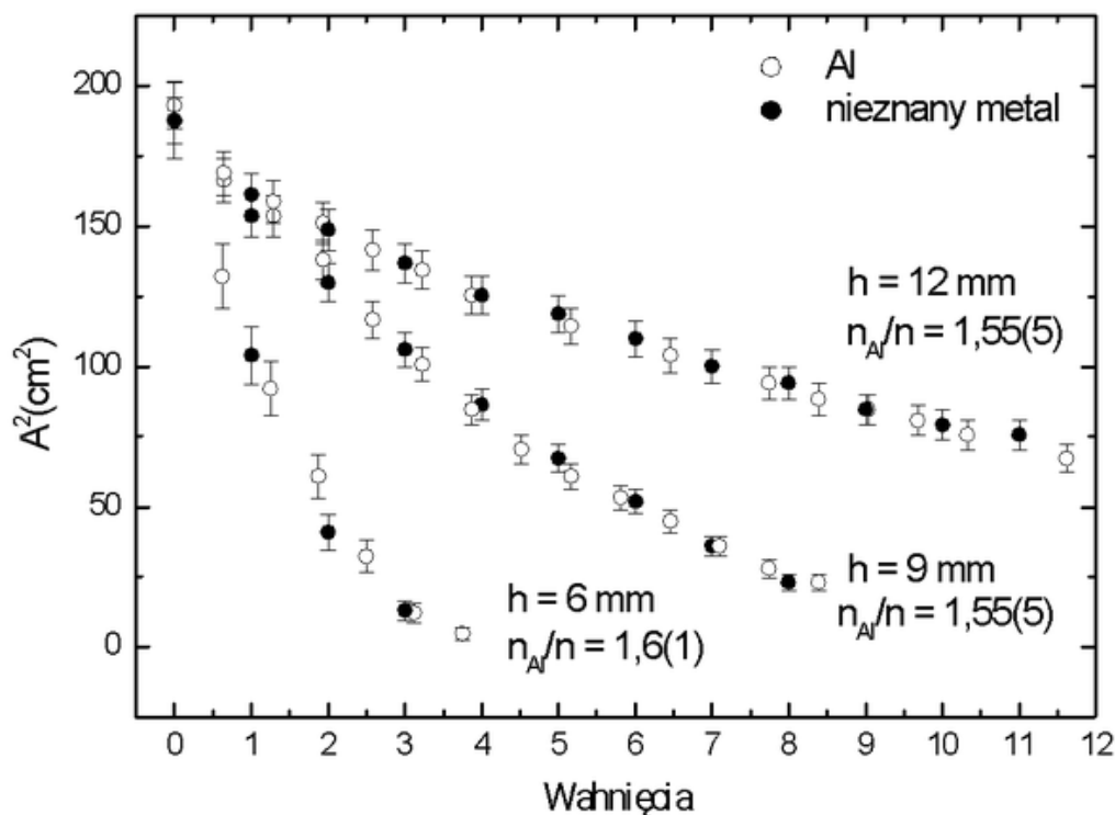
Rysunek 5: Wyniki pomiarów po przeskalowaniu dla różnych wysokości zawieszenia magnesu nad płytkami.
