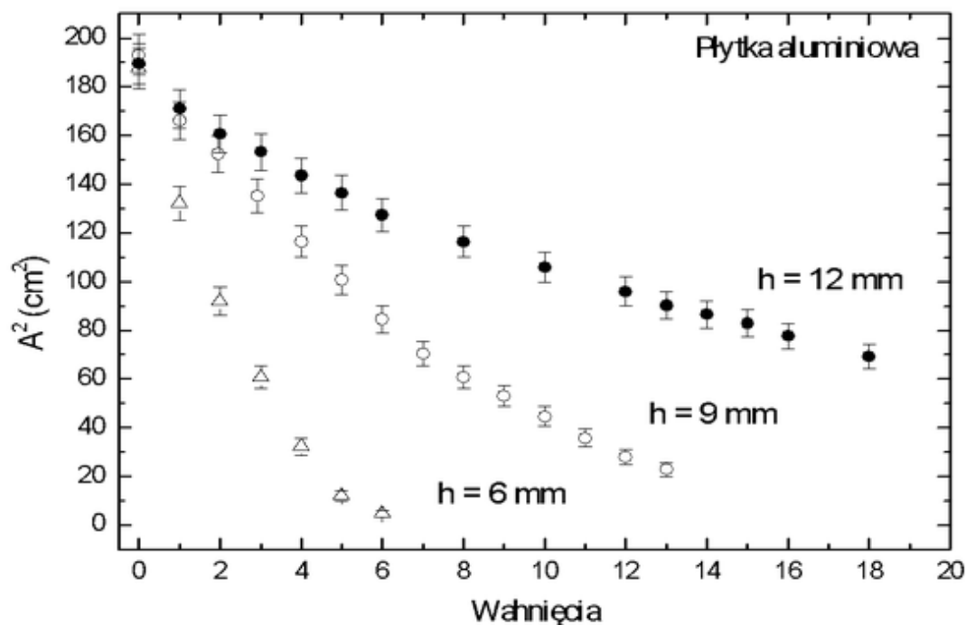
Rysunek 3: Pomiary amplitudy drgań wahadła z płytką w odległości h od jego najniższego położenia.
